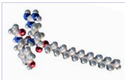
N-ацетил-Тирозил-Аргинил-О-гексадециловый эфир
